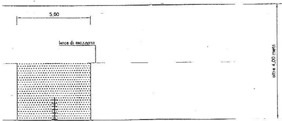
figura 8 scavo trasversale alla carreggiata
